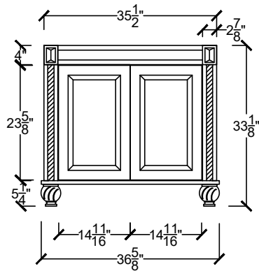
ANAV 3622 - - - -
