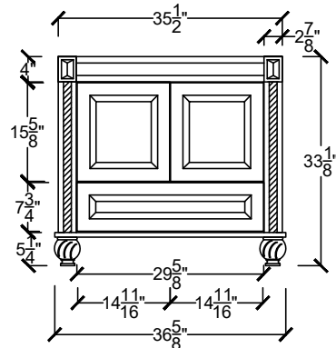
ANAV 3622 BD- - - -
