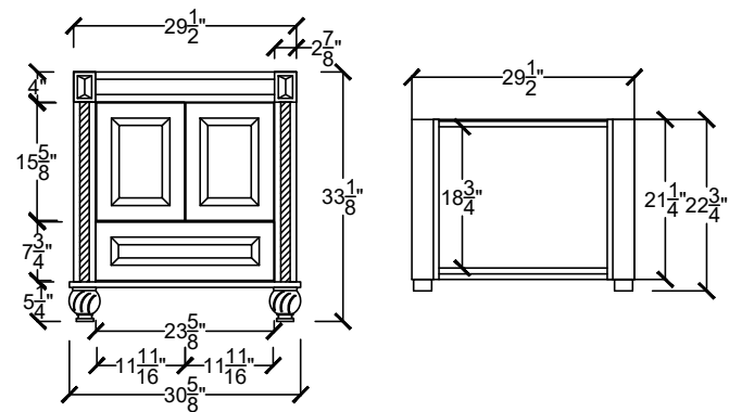
ANAV 3022 BD- - -
